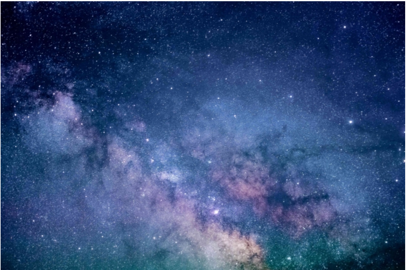
Galaxie
